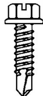
Sechskantkopf geschlitzt = DIN 7504L
